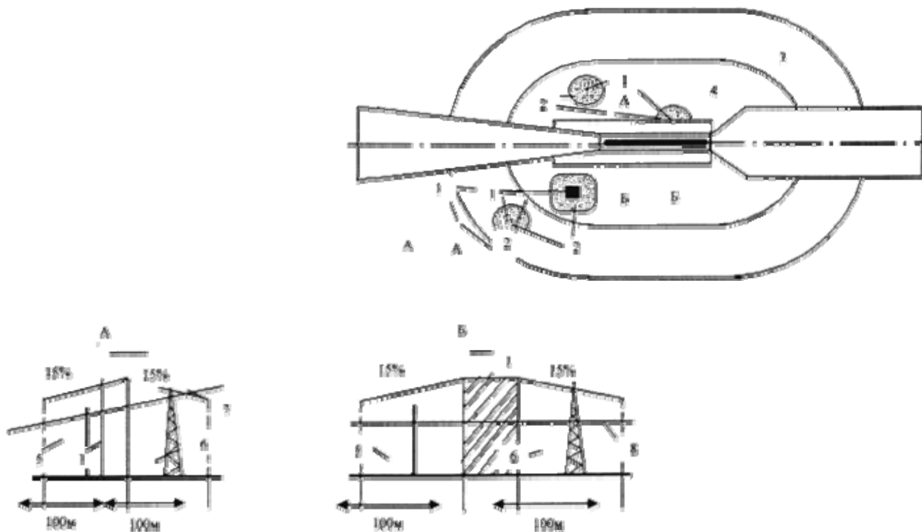
Рис.1. К образованию зоны "затенения" препятствиями, расположенными в пределах внутренней горизонтальной и конической поверхностей:
